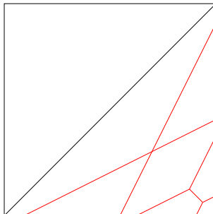
Figure 12: L'image pour les paires d'angles \{\varepsilon, 2\pi - \varepsilon\} , \{\eta, 2\pi - \eta\} ; ici \tilde{\mu} est surjective
