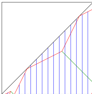
Figure 11: L'image pour les paires d'angles \{\frac{2\pi}{4}, -\frac{2\pi}{6}\} , \{\frac{2\pi}{5}, -\frac{2\pi}{7}\} (type D_{-+}^{+-} )
