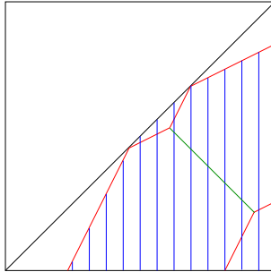
Figure 8: L'image pour les paires d'angles \{\frac{2\pi}{3}, -\frac{2\pi}{4}\} , \{\frac{2\pi}{5}, -\frac{2\pi}{6}\} (type C_{-+}^{+-} )
