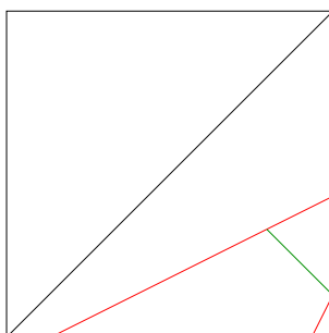
Figure 4: L'image pour les paires d'angles \{0, \frac{2\pi}{3}\} , \{0, \frac{8\pi}{5}\} (non convexe)
