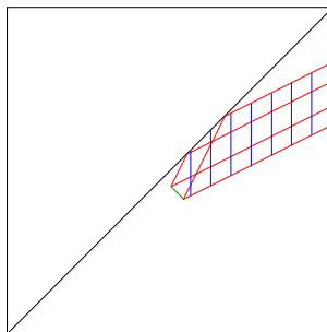
Figure 7: L'image pour les paires d'angles \{\frac{2\pi}{3}, \frac{2\pi}{4}\}, \{\frac{2\pi}{5}, \frac{2\pi}{6}\} (type C_{++}^{++} )
