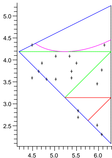
Figure 13: Groupes discrets dans le triangle des configurations pour p = 3
