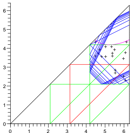
Figure 14: Groupes discrets et polygone de configurations pour p = 2, 3, \dots, 10
