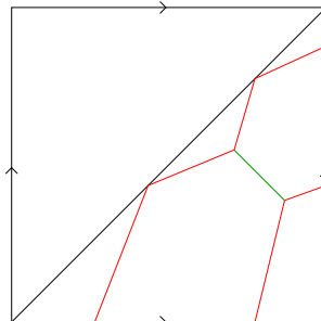
Figure 1: Une configuration de réductibles
