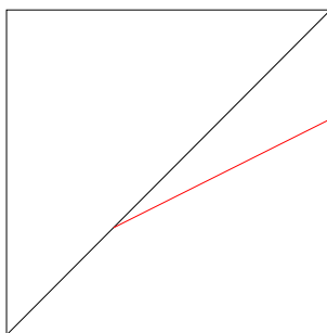
Figure 2: L'image pour les paires d'angles \{\frac{2\pi}{6}, \frac{2\pi}{6}\} , \{\frac{2\pi}{8}, \frac{2\pi}{8}\}
