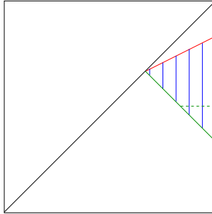
Figure 5: L'image pour les paires d'angles \{\frac{2\pi}{3}, \frac{4\pi}{3}\}, \{0, \frac{2\pi}{3}\} ; le segment en pointillés représente la famille \Gamma(3, t) de Mostow.
