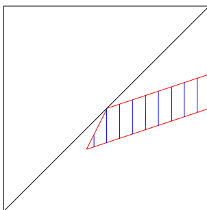
Figure 3: L'image pour les paires d'angles \{\frac{2\pi}{4}, \frac{2\pi}{6}\} , \{\frac{2\pi}{8}, \frac{2\pi}{8}\}
