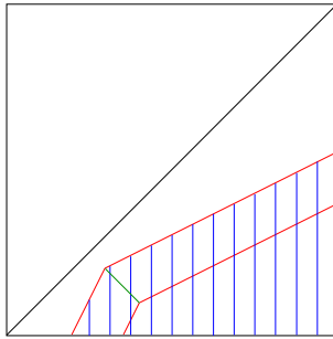
Figure 9: L'image pour les paires d'angles \{-\frac{2\pi}{10}, \frac{2\pi}{10}\} , \{\frac{4\pi}{10}, \frac{6\pi}{10}\} (type C_{-+}^{-+} )
