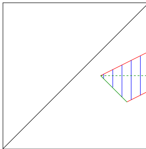
Figure 6: L'image pour les paires d'angles \{\frac{2\pi}{3}, \frac{4\pi}{3}\}, \{0, \frac{2\pi}{6}\} ; le segment en pointillés représente la famille \Gamma(6, t) de Mostow.
